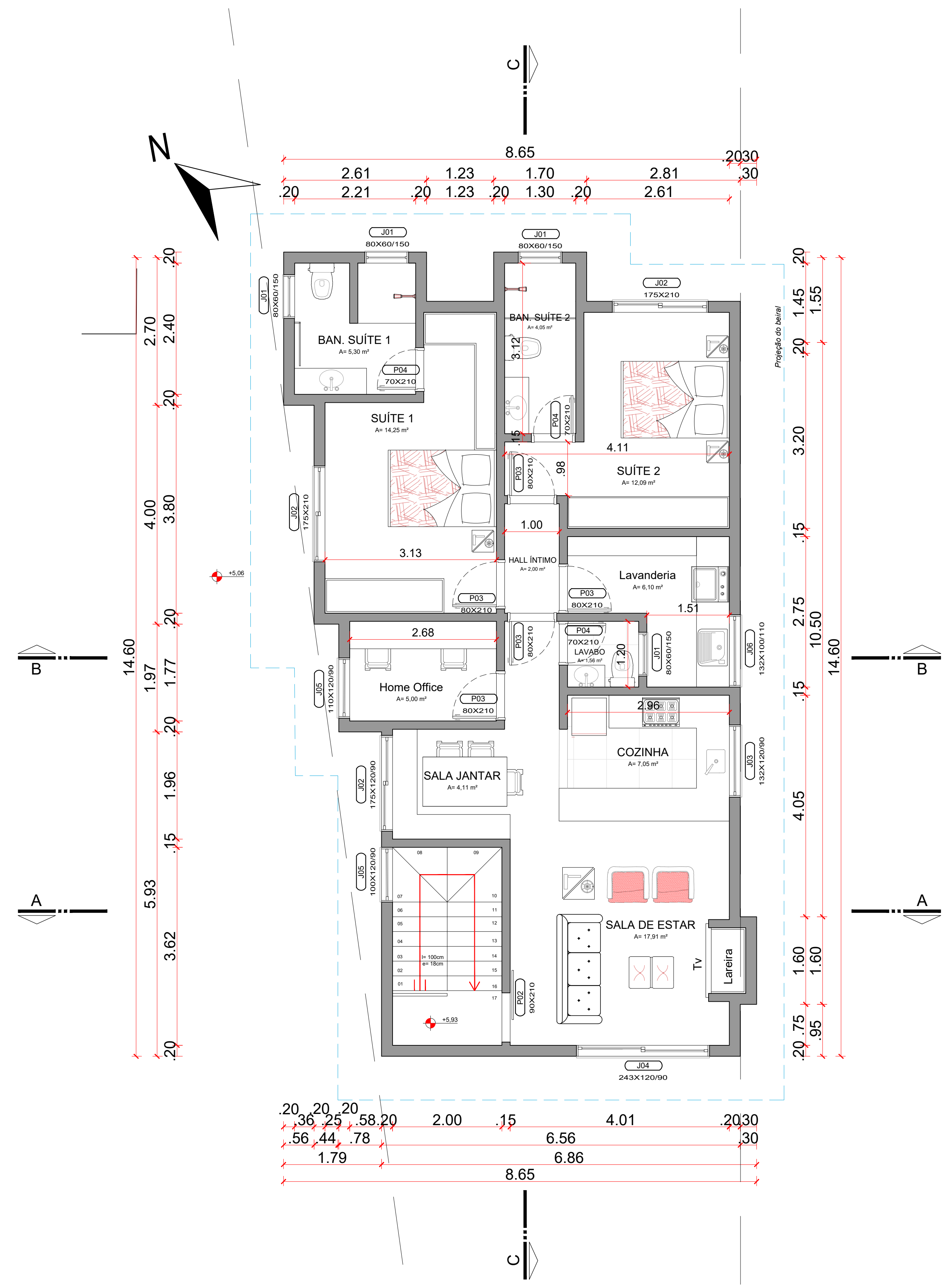
PLANTA BAIXA PRIMEIRO PAVIMENTO Área Total: 104,77m²
