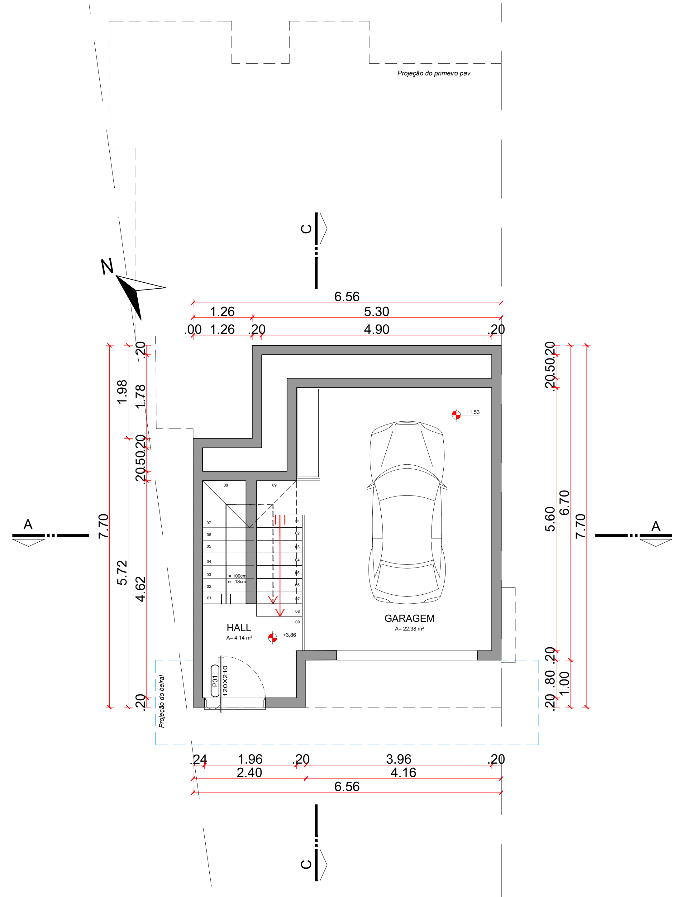
PLANTA BAIXA TÉRREO Área Total: 43,85m²
